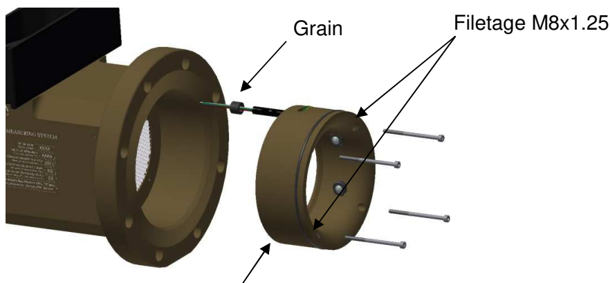
Entretoise 2 DLA équipée (code 2319)
